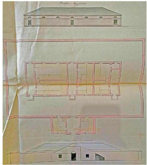
Мал. 2 План тюремних замків в Херсоні, Тирасполі, Ольвіополі та Єлизаветграді 107
